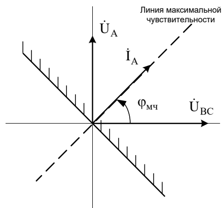
Рисунок 5 – Векторная диаграмма токов и напряжений, подаваемых на ИО направления мощности терминала БЭ2502А0103.
