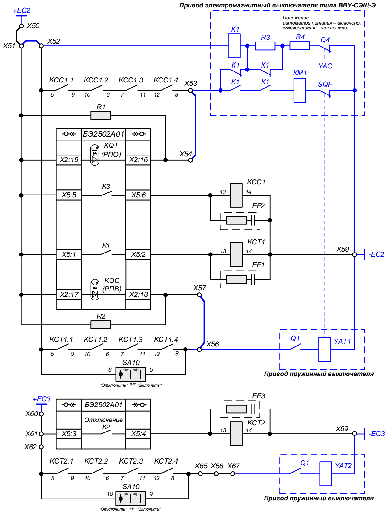
Рисунок 8 - Схема подключения выключателя ВВУ-СЭЦ-ЭЗ-10 к клеммам комплекта 01
