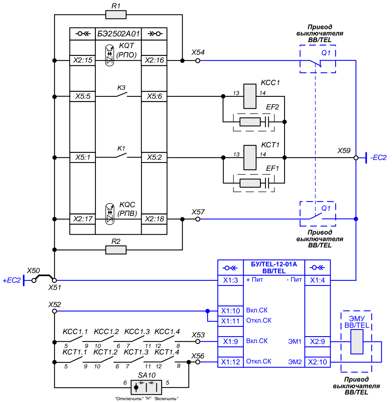
Рисунок 9 - Схема подключения выключателя ВВ/TEL-10 к клеммам комплекта 01
