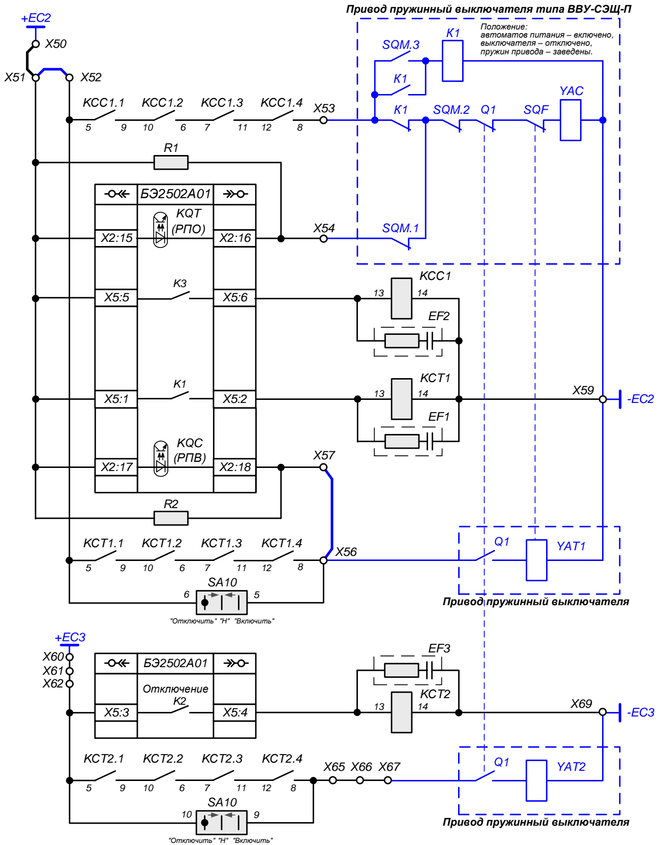
Рисунок 7 - Схема подключения выключателя ВВУ-СЭЩ-ПЗ-10 (ВБП-10-20, ВВЭ-М, ВБЭК) к клеммам комплекта 01
